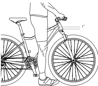
Afb. 1/14 Inch-afstand
