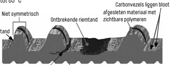
Afb. 3/28 Riemslijtage bron Gates
