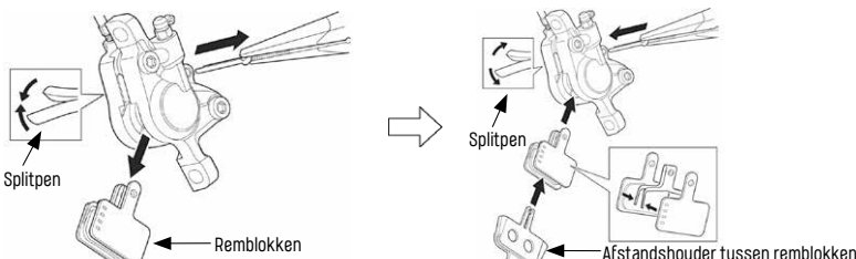
Afb. 3/20 Bron Shimano
