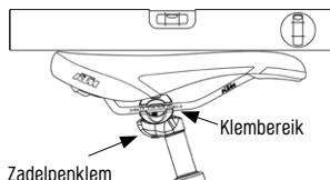
Afb. 4/15 Zadelmontage
