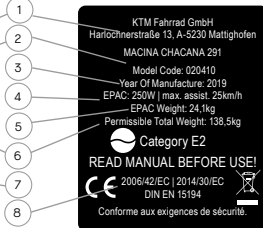
Afb. 2/10 EPAC-sticker
