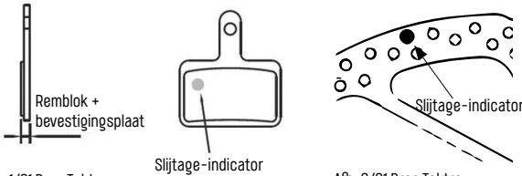
Afb. 1/21 Bron Tektro
