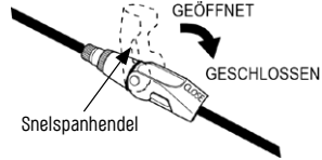
Afb. 4/19 Bron Shimano
