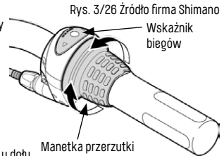
Manetka przerezutek
