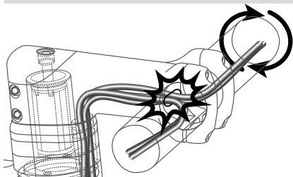
Rys. 1/16 Wewnętrznie poprowadzone przewody hamulcowe i linki przerzutek
