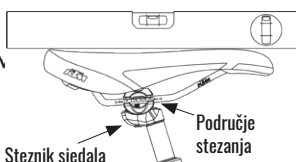
Sl. 4/23 Montaža sjedala
