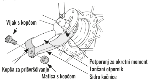
Sl. 3/29 Sidro kočnice, izvor: Shimano
