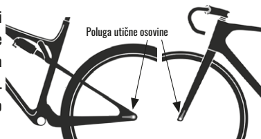
Sl. 2/38 Utična osovina KTM
