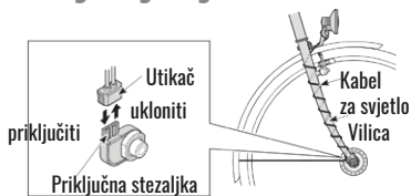
Sl. 2/49 Priključna stezaljka dinamo-glavčine Izvor: Shimano
