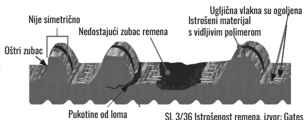
Sl. 3/36 Istrošenost remena, izvor: Gates
