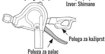
Sl. 4/31 Jedinica poluge mjenjača za stražnji mjenjač Izvor: Shimano
