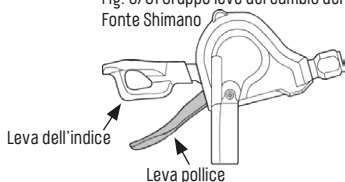
Fig. 3/31 Gruppo leve del cambio deragliatore Fonte Shimano
