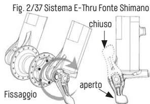
Fig. 2/37 Sistema E-Thru Fonte Shimano
