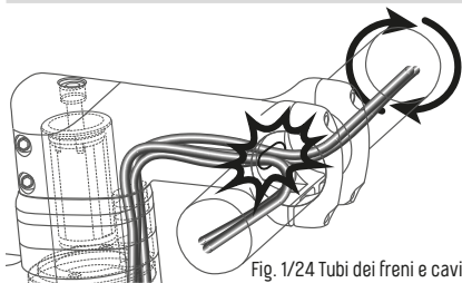
Fig. 1/24 Tubi dei freni e cavi del cambio installati internamente
