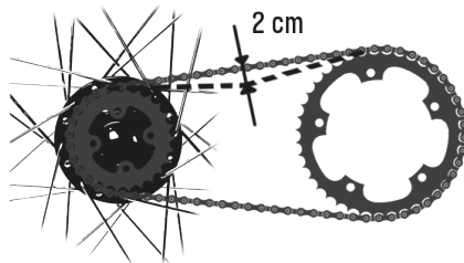
Fig. 4/29 Tensione catena
