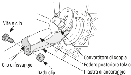
Fig. 3/29 Piastra di ancoraggio Fonte Shimano
