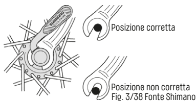
Fig. 3/38 Fonte Shimano
