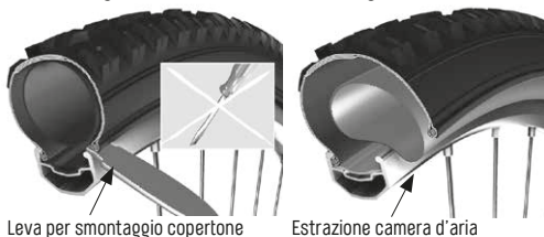
Leva per smontaggio copertone
