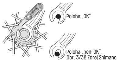
Seřizovací matice
