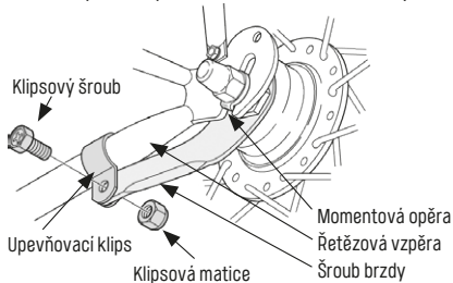
Obr. 3/29 Šroub brzdy Zdroj Shimano
