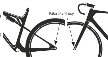
Obr. 2/38 Pevná osa KTM
