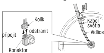
Obr. 2/49 Konektor nábojového alternátoru Zdroj: Shimano
