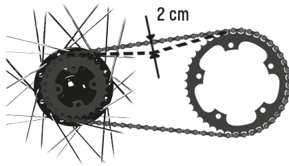
Obr. 4/29 Napětí řetězu
