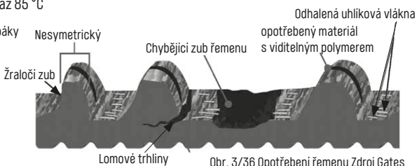
Obr. 3/36 Opotřebení řemenu Zdroj Gates
