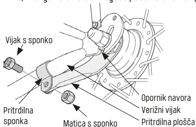
Slika 3/29 Pritrdilna ploščica vir Shimano
