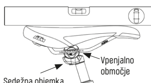
Sedežna objemka Slika 4/23 Namestitvev sedeža
