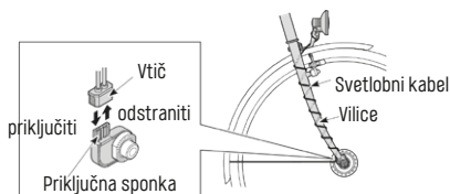
Slika 2/49 Priključna sponka dinama pesta Vir: Shimano
