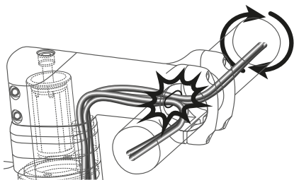
Slika 1/24 Pletenice zavor in prestavna potezala, napeljeni v notranjosti
