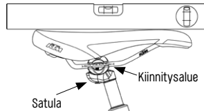
Kuva 4/15 Satulan asennus
