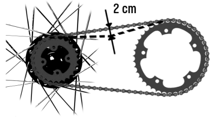
Kuva 4/21 Ketjun kireys
