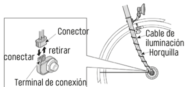
Fig. 2/49 Terminal de conexión de la dinamo de buje Fuente: Shimano
