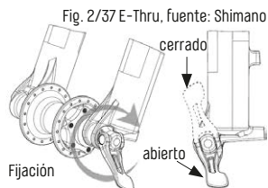
Fig. 2/37 E-Thru, fuente: Shimano
