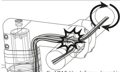
Fig. 1/24 Cables de freno y de cambios tendidos internamente
