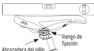
Fig. 4/23 Montaje del sillín
