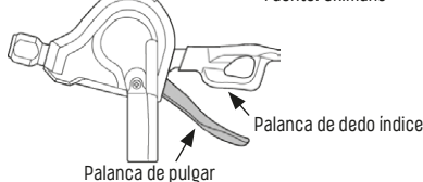
Fig. 4/31 Unidad de cambio - Desviador trasero
