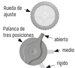
Fig. 1/46 Índice de compresión, fuente: Fox
