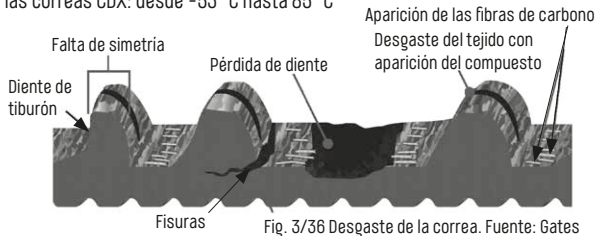
Fig. 3/36 Desgaste de la correa. Fuente: Gates
