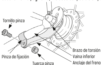
Fig. 3/29 Anclaje del freno. Fuente: Shimano
