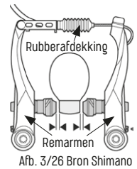
Afb. 3/26 Bron Shimano
