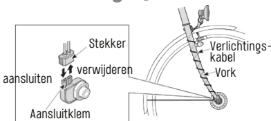
Afb. 2/49 klem naafdynamo Bron: Shimano
