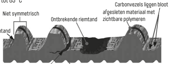
Afb. 3/36 Riemslijtage bron Gates
