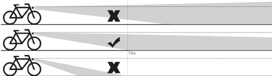
Afb. 1/49 lichtinstelling
