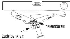
Afb. 4/23 Zadelmontage
