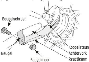
Afb. 3/29 Reactiearm bron Shimano
