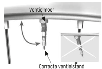
Afb. 2/43 bron Schwalbe
