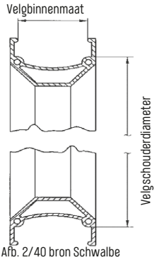
Afb. 2/40 bron Schwalbe
