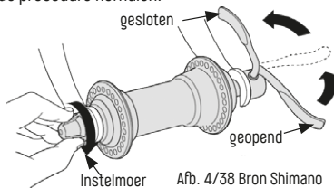
Afb. 4/38 Bron Shimano
