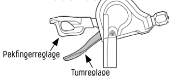
Fig. 3/23 Växelhandtagsenhet kedjeväxel
