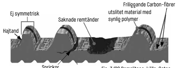
Fig. 3/28 Remslitage, källa: Gates
