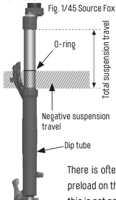
Fig. 1/45 Source Fox
