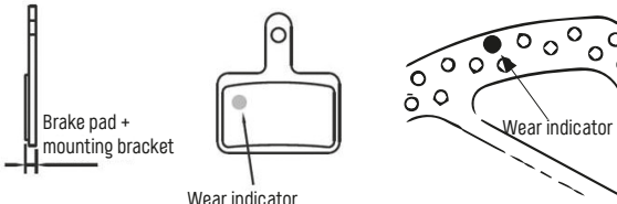
Fig. 1/29 Source Tektro
