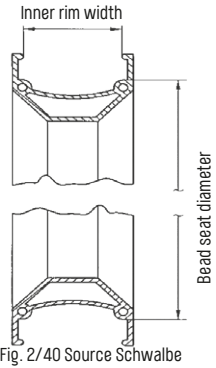
Fig. 2/40 Source Schwalbe
