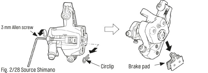
Fig. 2/28 Source Shimano
