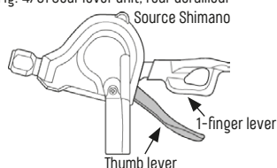
Fig. 4/31 Gear lever unit, rear derailleur Source Shimano
