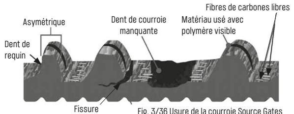
Fig. 3/36 Usure de la courroie Source Gates
