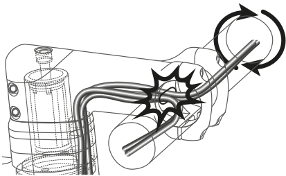
Fig. 1/24 Conduites de freinage et les câbles de vitesse internes
