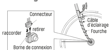
Fig. 2/49 Borne de connexion Moyeu dynamo Source : Shimano
