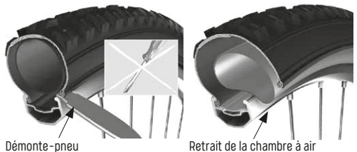
Fig. 4/42 Source Schwalbe
