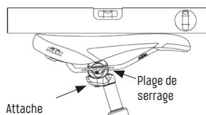
Fig. 4/23 Montage de la selle
