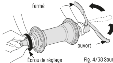
Fig. 4/38 Source Shimano
