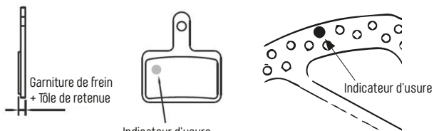
Fig. 1/29 Source Tektro
