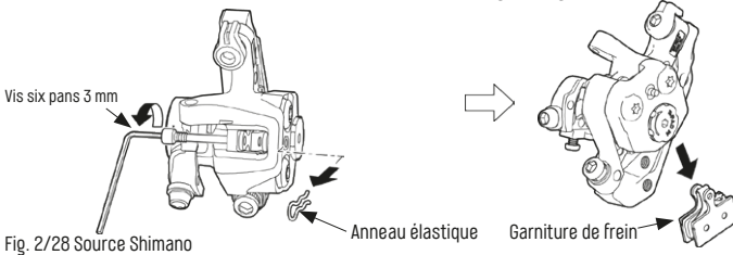
Fig. 2/28 Source Shimano
