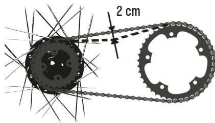
Εικ. 4/29 Προένταση αλυσίδας
