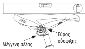
Εικ. 4/23 Εγκατάσταση σέλας
