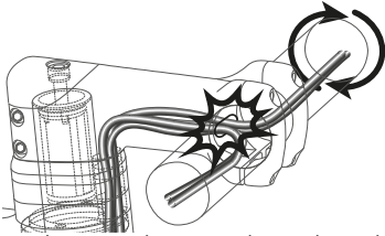
Εικ. 1/24 εσωτερικά εγκατεστημένοι σωλήνες φρένων και ντίζες αλλαγής ταχυτήτων
